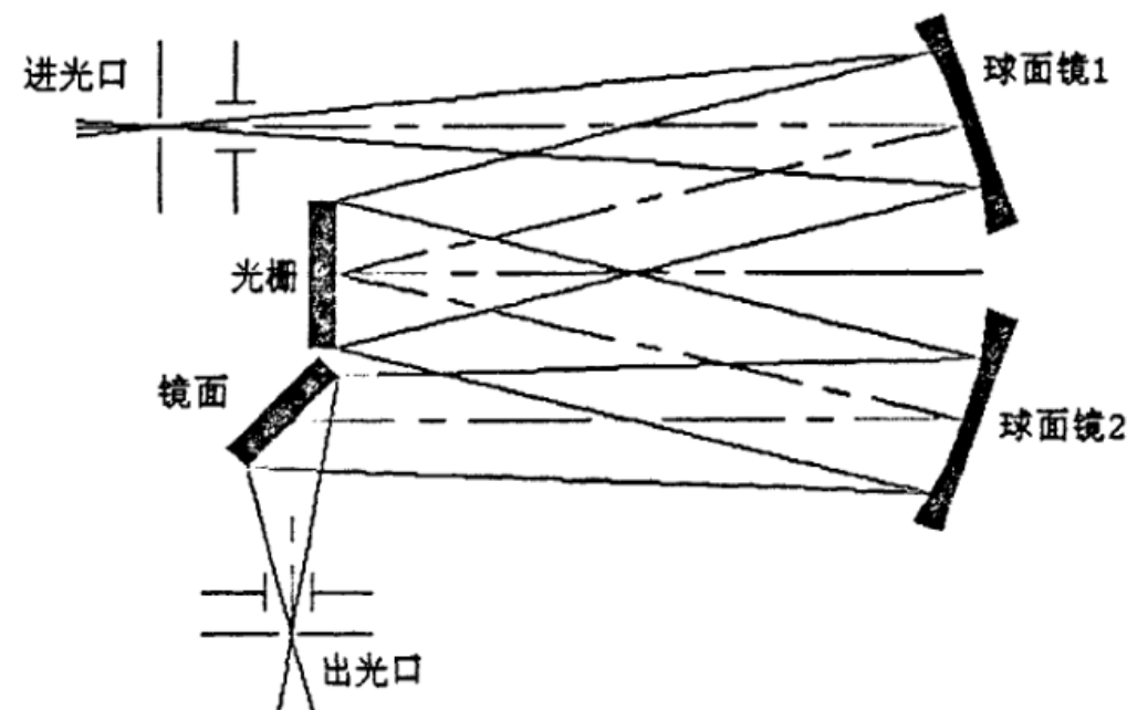
(车尼尔-特纳 (Czerny-Turner)) 光栅单色仪
